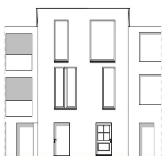
VOORGEVEL / ARCHICAD
